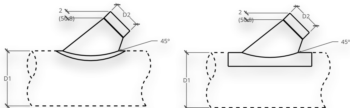
Contorno de Brida
